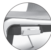
Reihenverbindung paniksicher zertifiziert nach DIN EN14703:2007 anti-panic ganging device in accordance with DIN EN14703:2007
